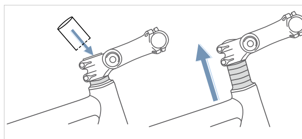
Figura 81: Aumento de la potencia Ahead mediante el montaje de anillos distanciadores (reductores)
