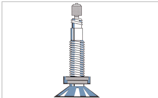
Figura 16: Válvula Presta
