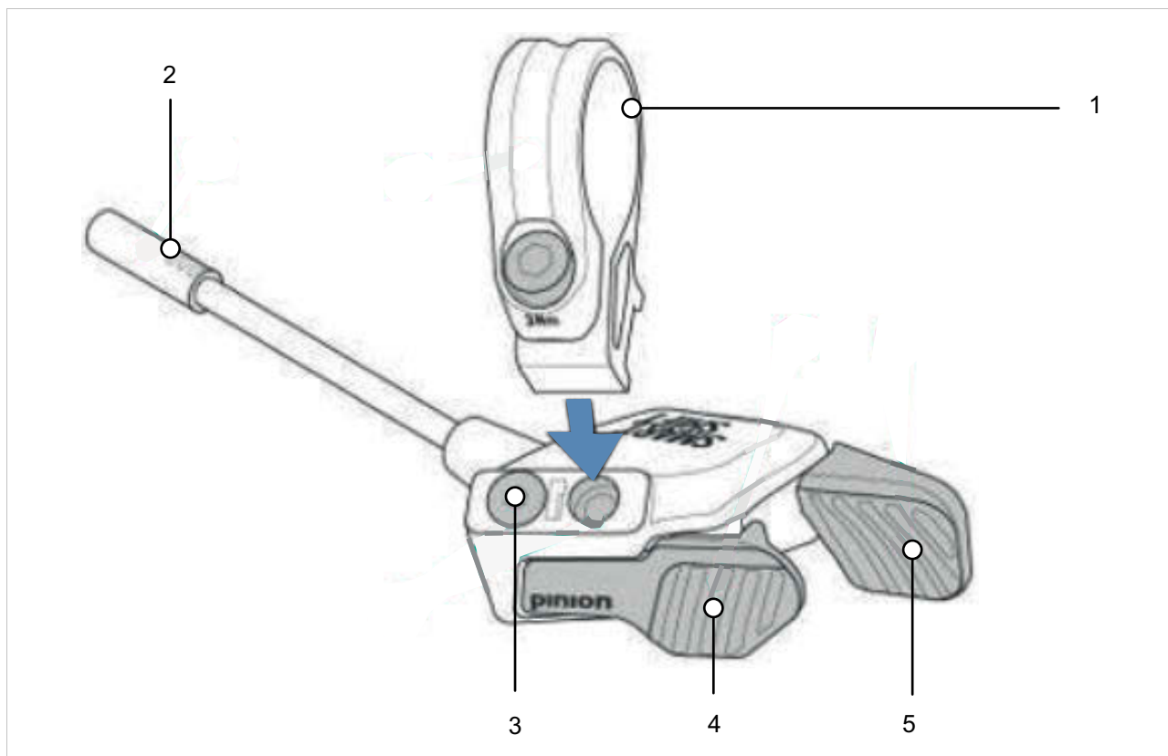
Figura 51: Estructura Pinion E-Trigger TE1
