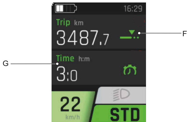
Figura 44: Vista general de la VISUALIZACIÓN PRINCIPAL TRIP
