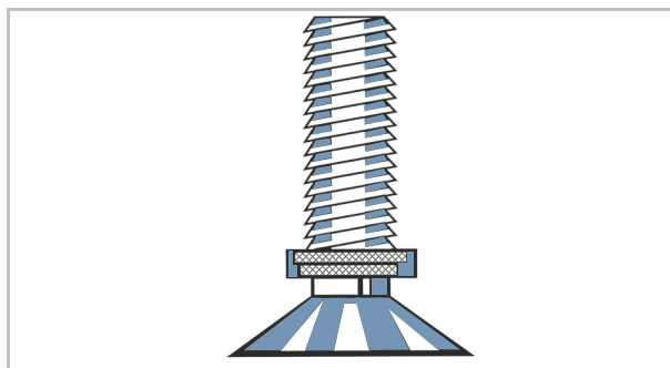
Figura 17: Válvula Schrader
