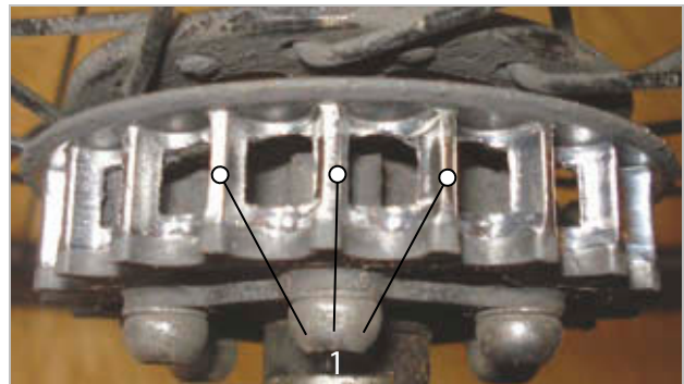
Figura 144: Fotografía de ejemplo de un perfil dentado desgastado
