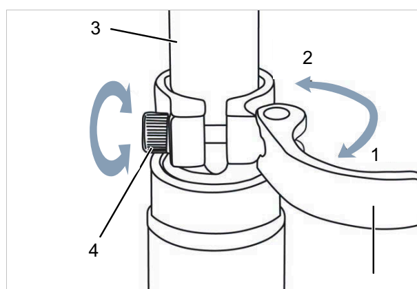
Figura 72: Apertura del cierre rápido de la tija de sillín
