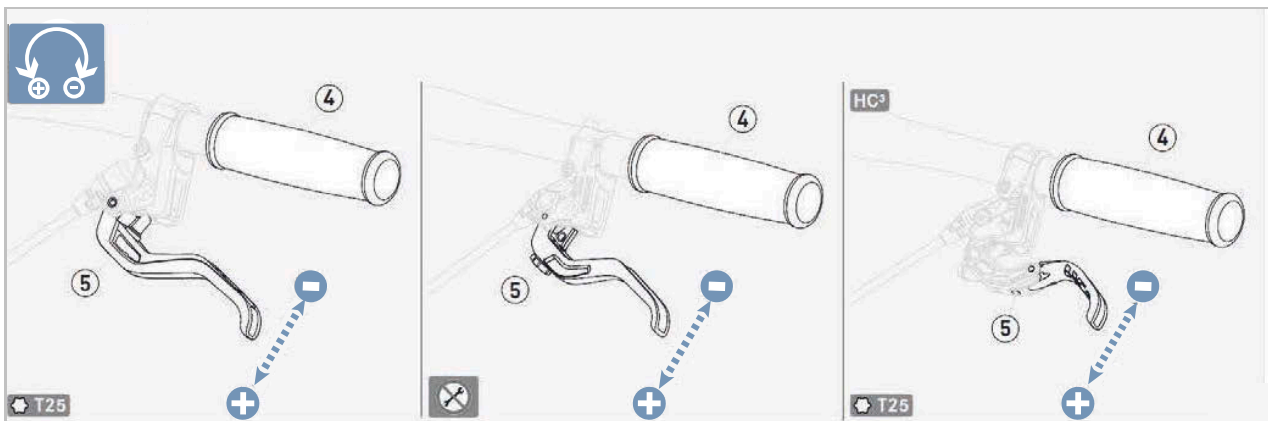
Figura 91: Ajuste del ancho de agarre del freno de mano con freno de disco MAGURA
